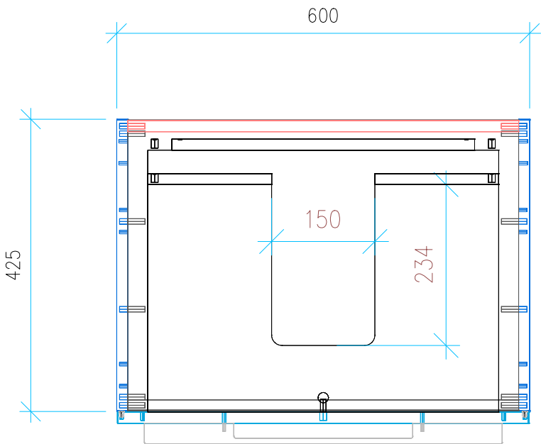
Ansicht 2 / Draufsicht
