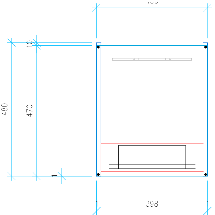
Ansicht 4 / Vorderansicht
