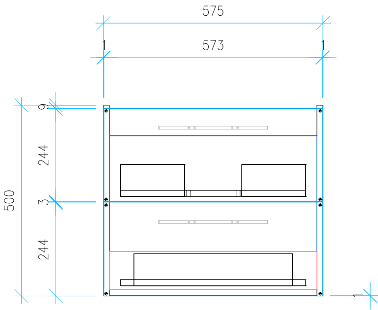
Ansicht 4 / Vorderansicht
