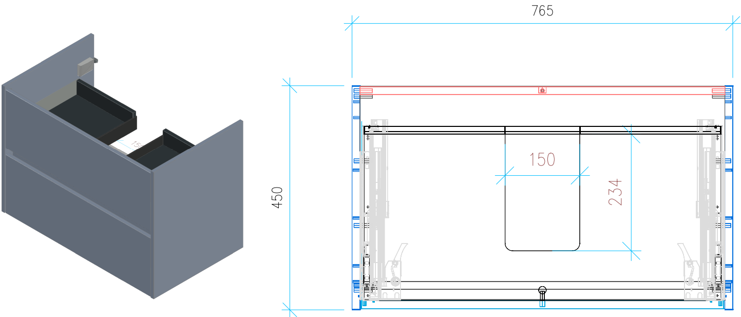
Ansicht 1 / 3D
