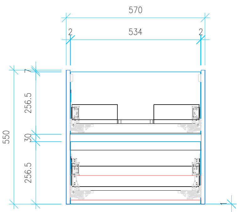
Ansicht 4 / Vorderansicht
