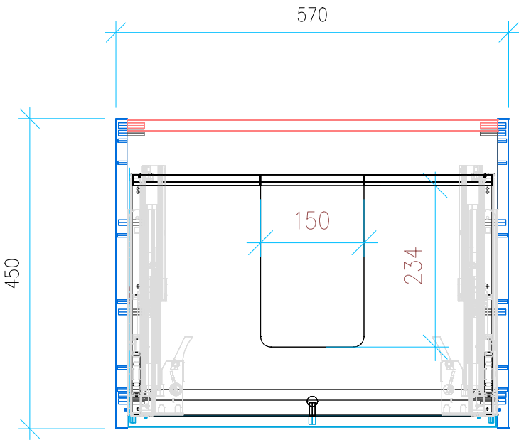
Ansicht 2 / Draufsicht
