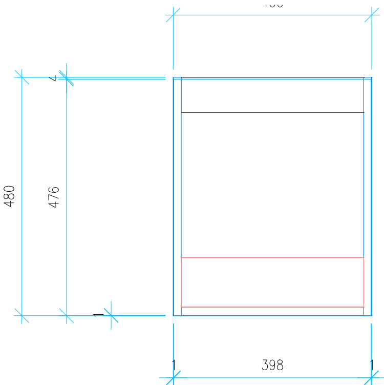
Ansicht 4 / Vorderansicht
