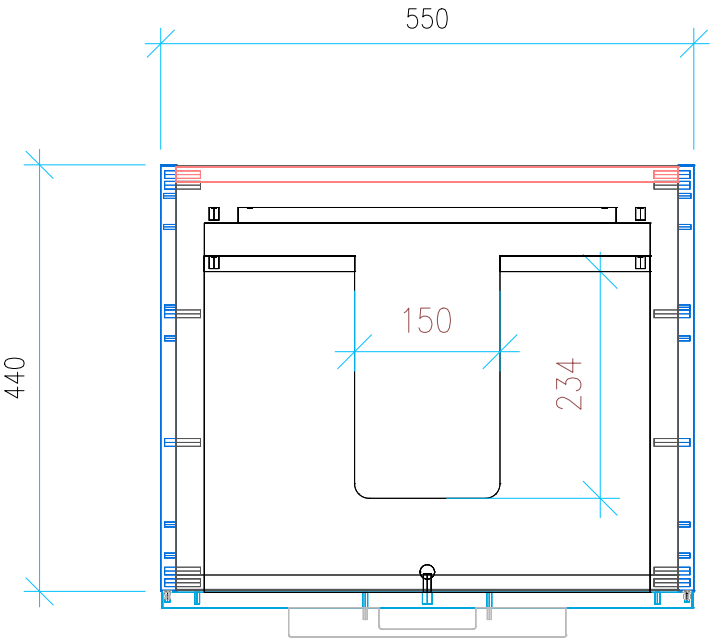
Ansicht 2 / Draufsicht
