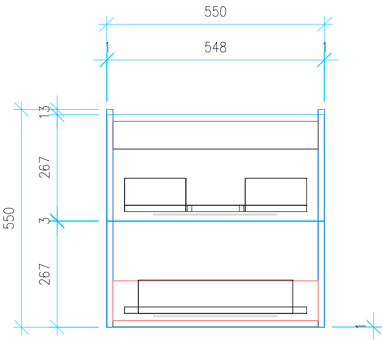
Ansicht 4 / Vorderansicht
