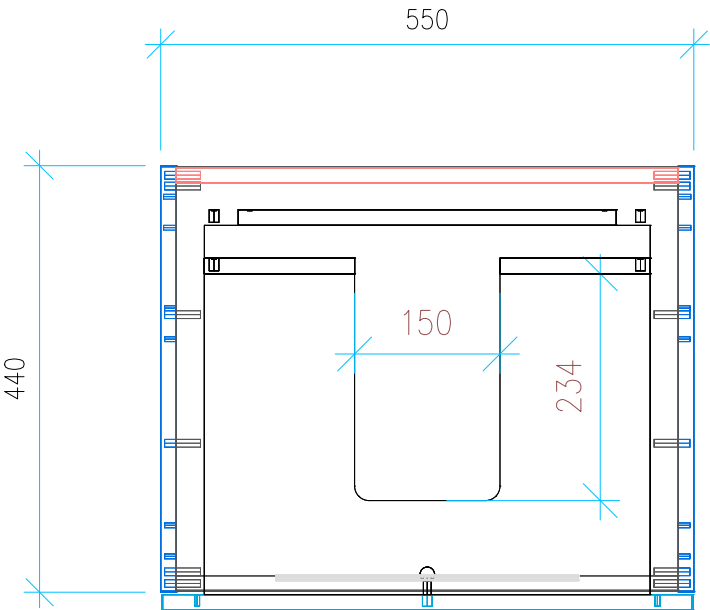
Ansicht 2 / Draufsicht
