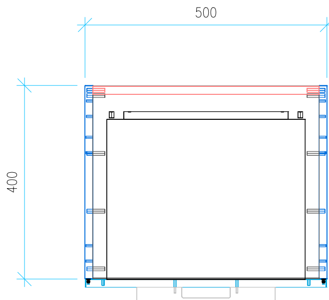
Ansicht 2 / Draufsicht
