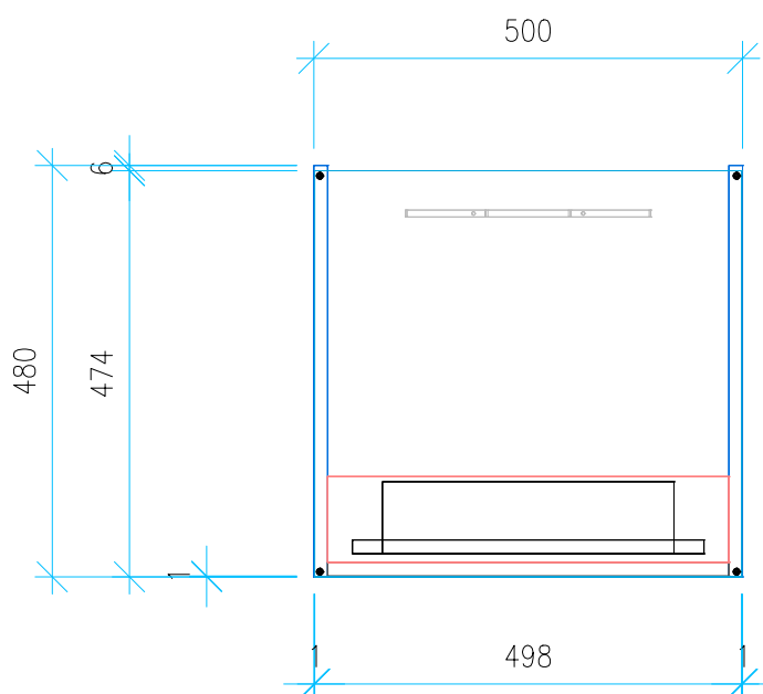
Ansicht 4 / Vorderansicht
