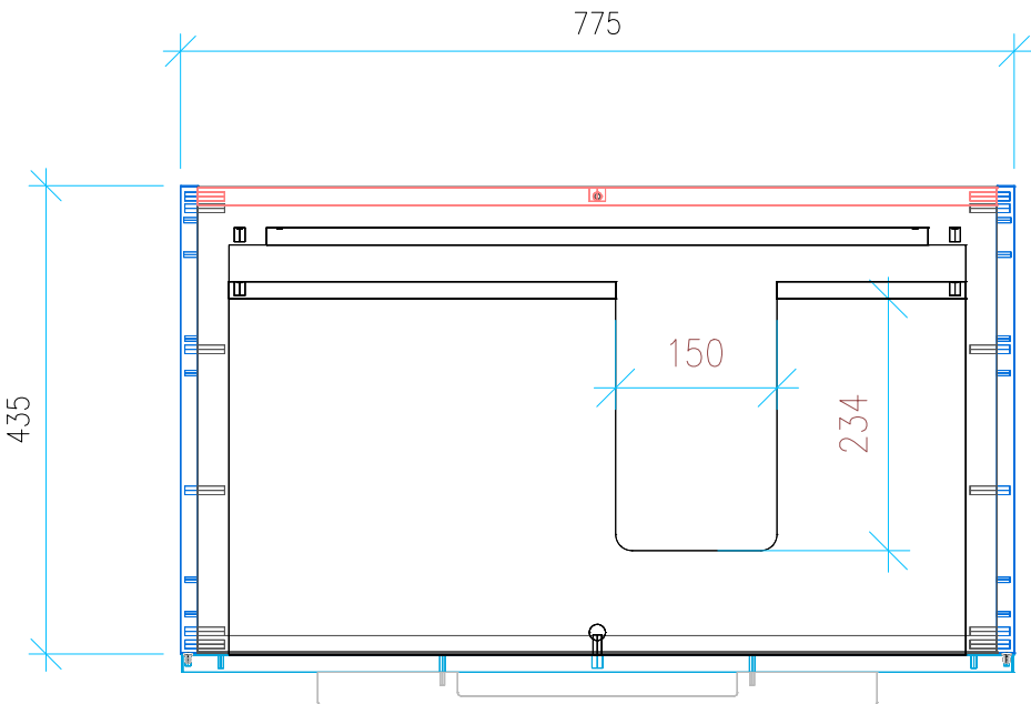
Ansicht 2 / Draufsicht
