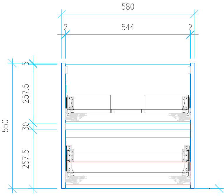
Ansicht 4 / Vorderansicht
