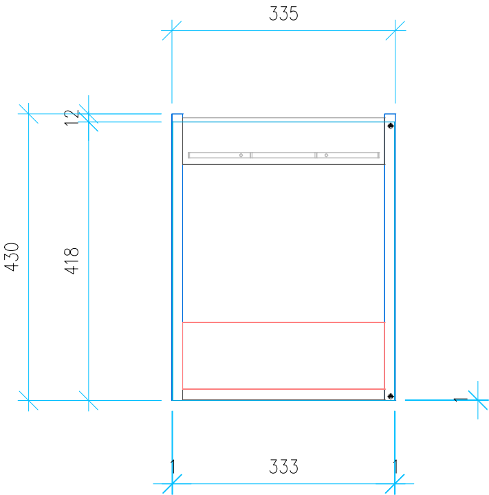
Ansicht 4 / Vorderansicht
