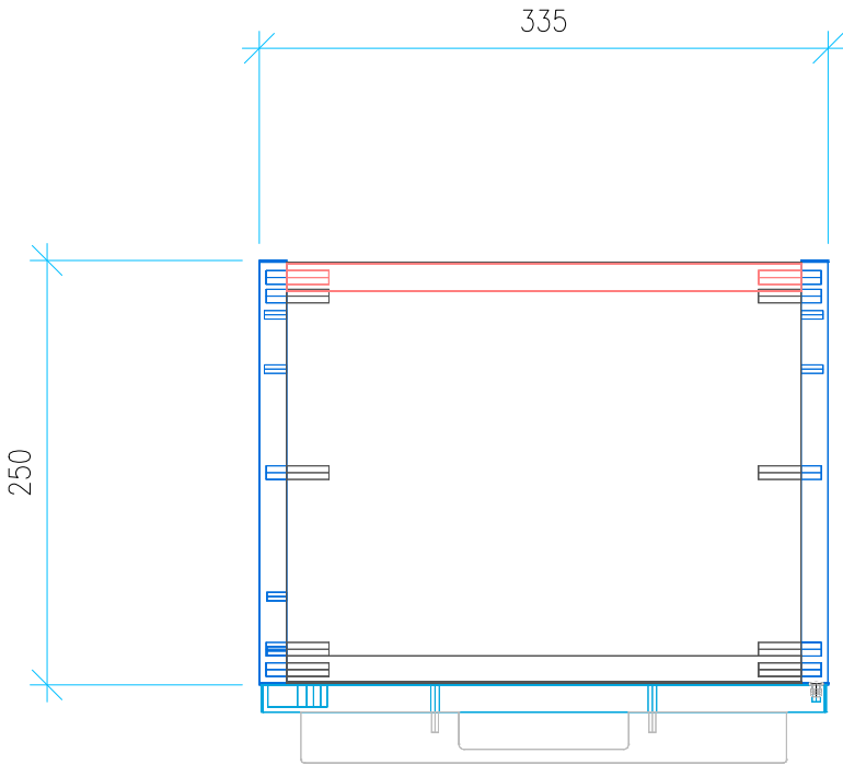
Ansicht 2 / Draufsicht
