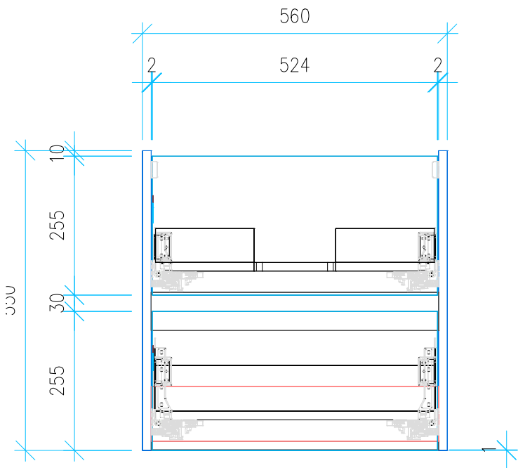
Ansicht 4 / Vorderansicht
