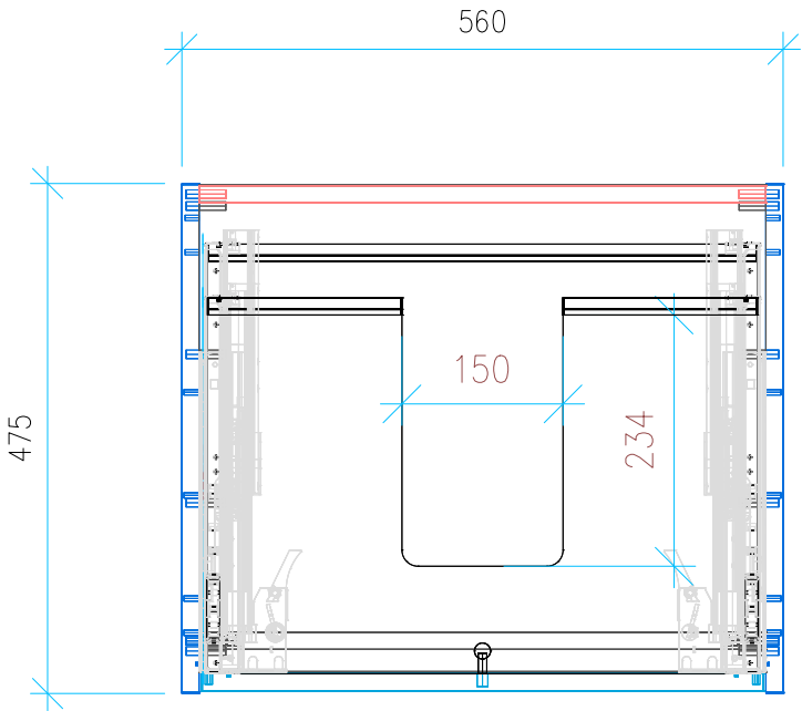
Ansicht 2 / Draufsicht
