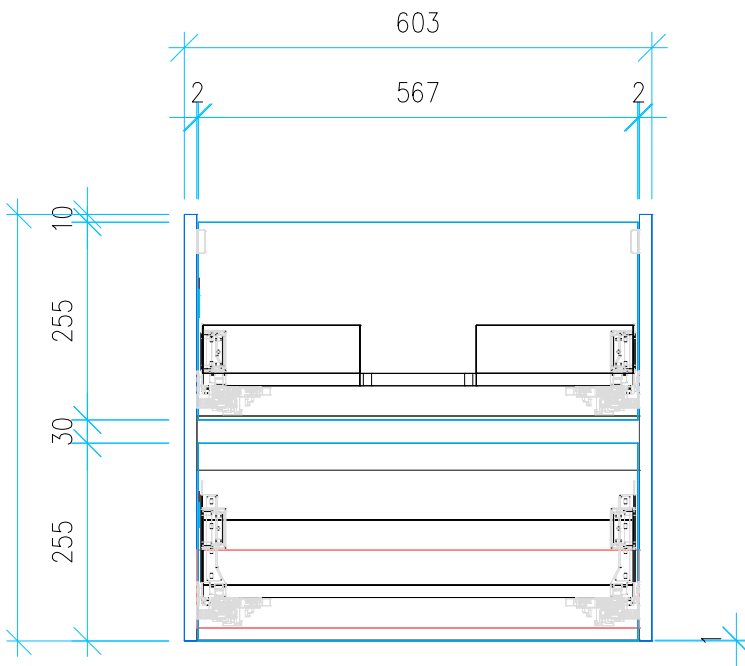
Ansicht 4 / Vorderansicht
