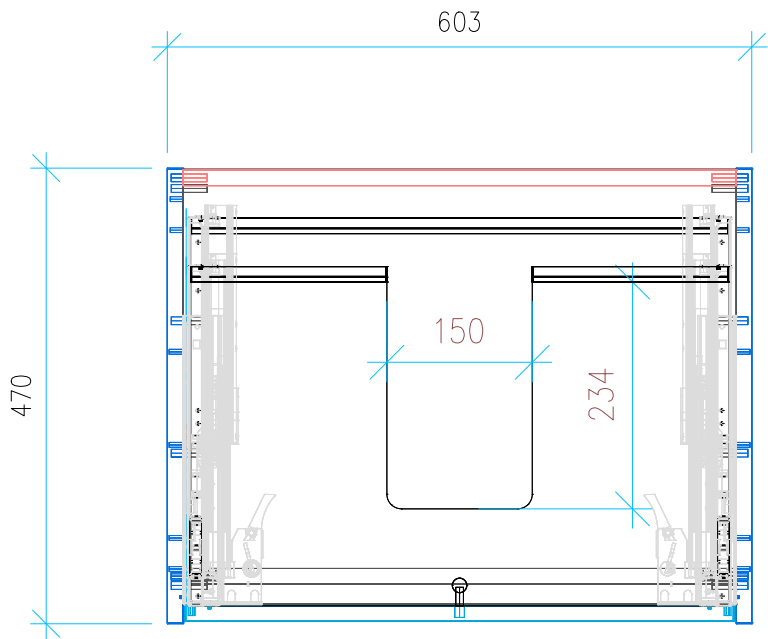
Ansicht 2 / Draufsicht
